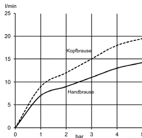
Diagram przepływu
