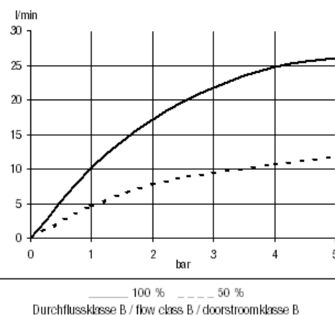
Diagram przepływu
