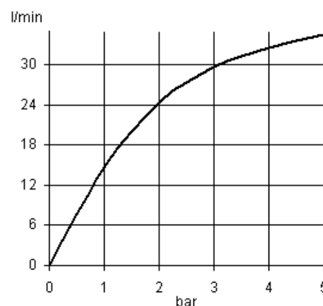
Diagram przepływu
