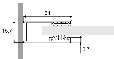
Przekrój profilu ścianki Wall profile cross-section Stěnové profily průřez
