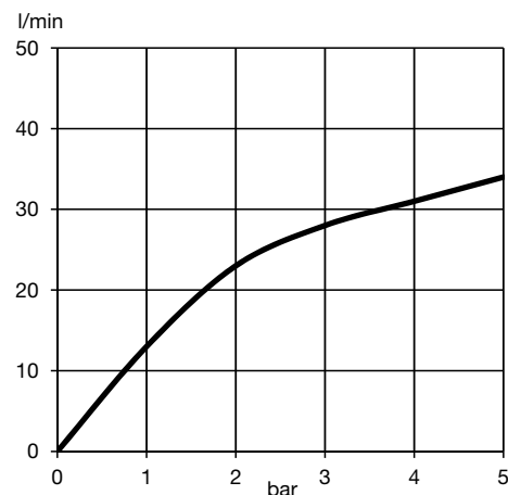
Diagram przepływu
