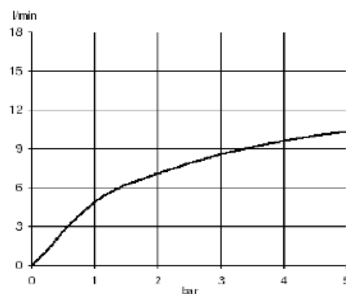
Diagram przepływu
