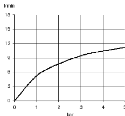
Diagram przepływu
